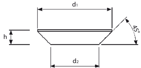
Geometrie Senkskopf bei Ausführung SZ-SK.
