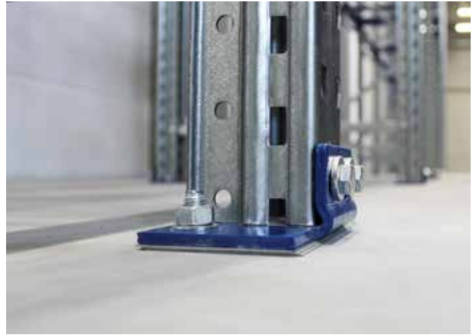
Bolzenanker BZ3
