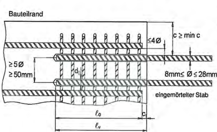
Bild B1: eingemörtelte Bewehrungsstäbe
